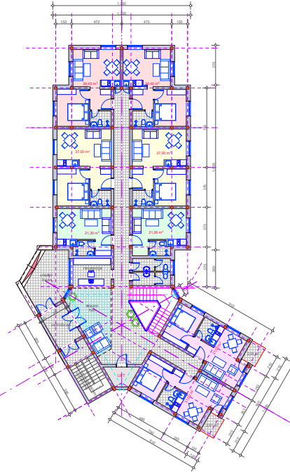
PRIZEMLJE 8 apartmana (2+6) BRGP=474m 2
