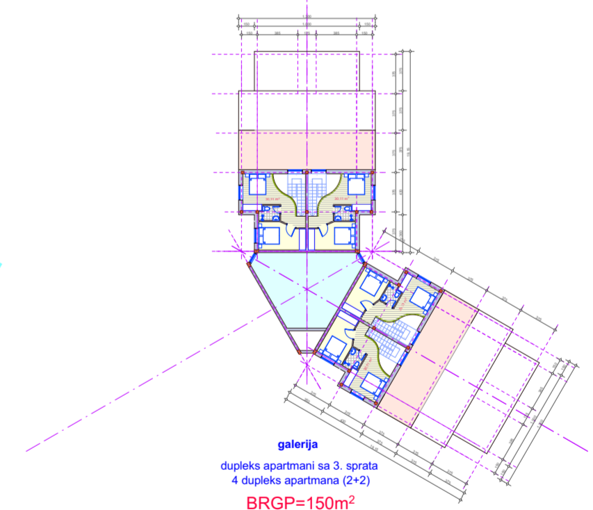
OBJEKAT "US-3." UGAONI SIMETRIČNI (P+3) (5+5)
