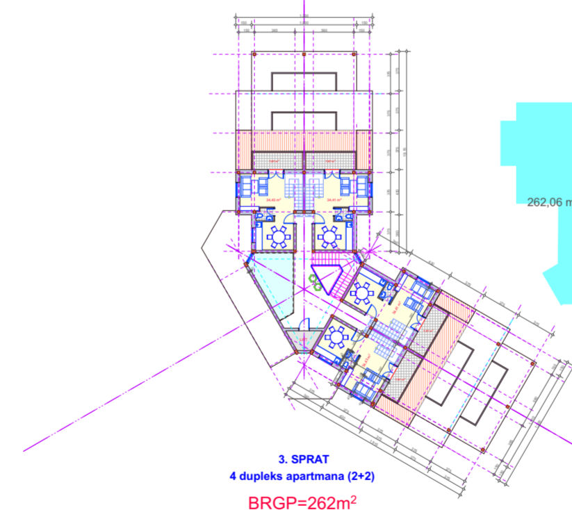
OBJEKAT "US-3." UGAONI SIMETRIČNI (P+3) (5+5)
