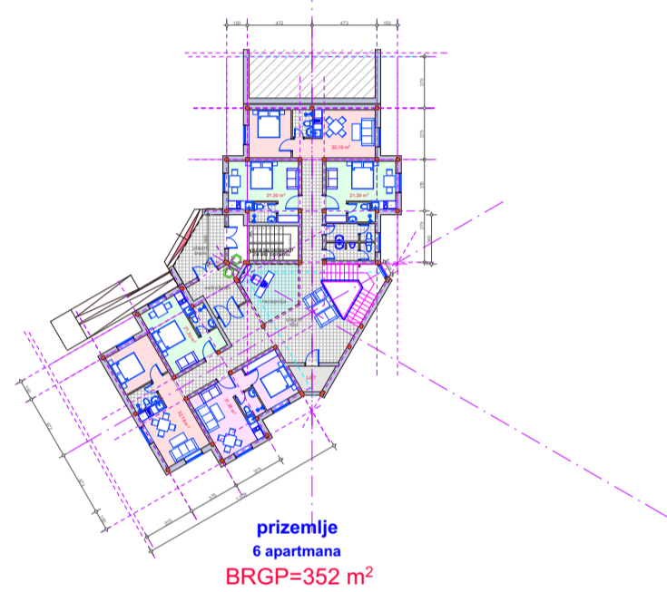
OBJEKAT "US-2" - ugaoni simetrični (P+2)
