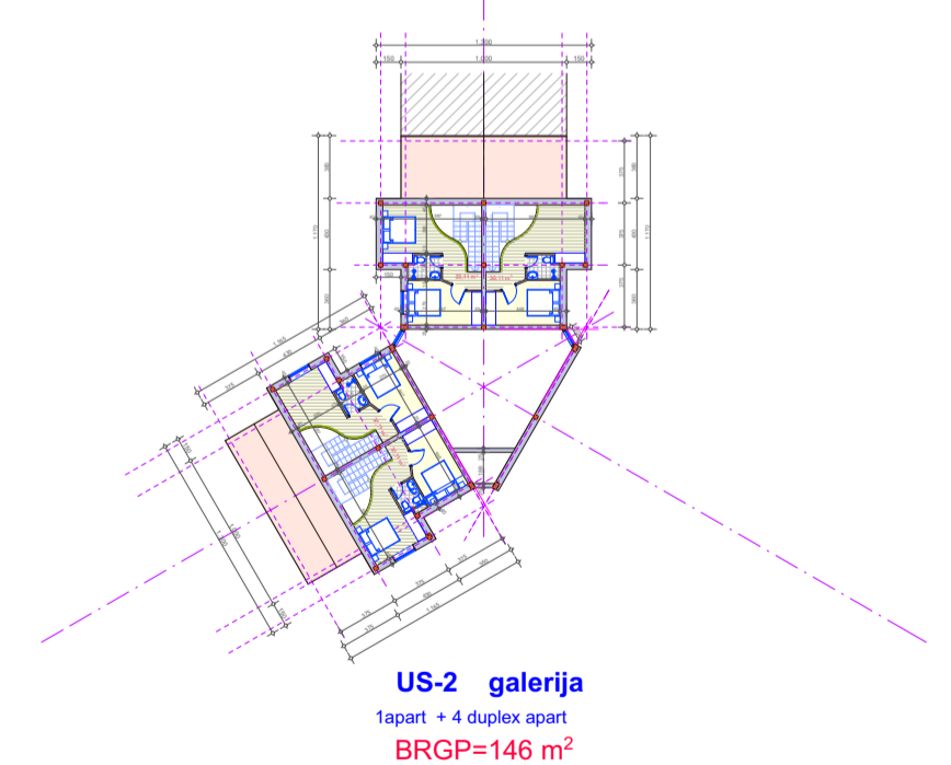
OBJEKAT "US-2" - ugaoni simetrični (P+2)
