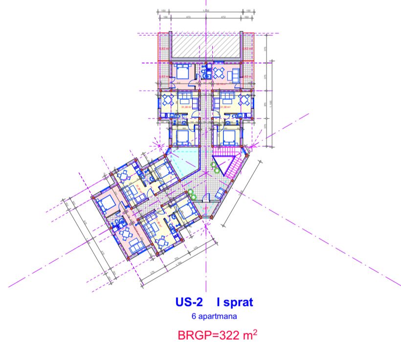
OBJEKAT "US-2" - ugaoni simetrični (P+2)
